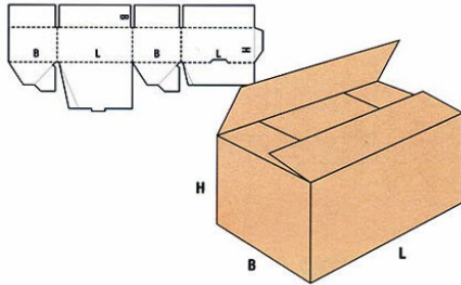
FEFCO 701
