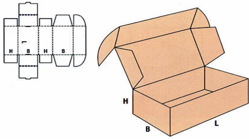
FEFCO 470
